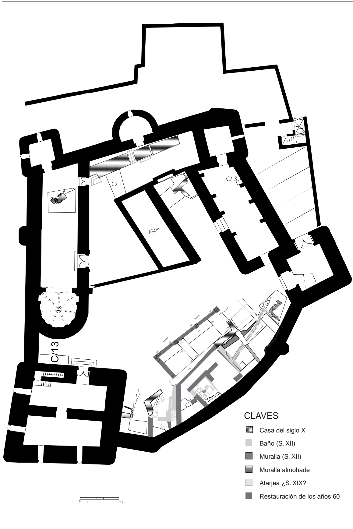
Fig. 1. Planta general del castillo
