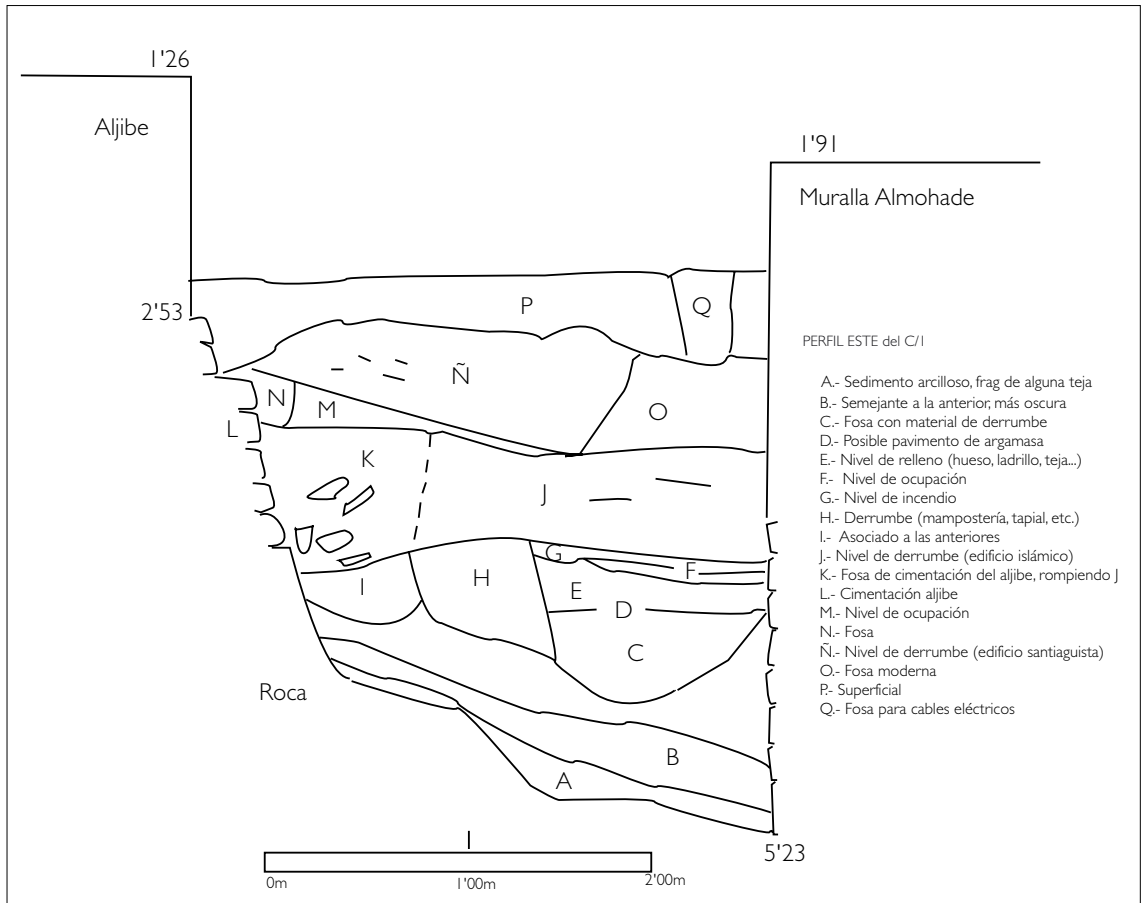
Fig. 4. Perfil entre el aljibe santiagoista y la muralla almohade
