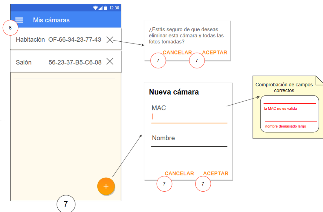
Ilustración 36: Mis cámaras del Storyboard
