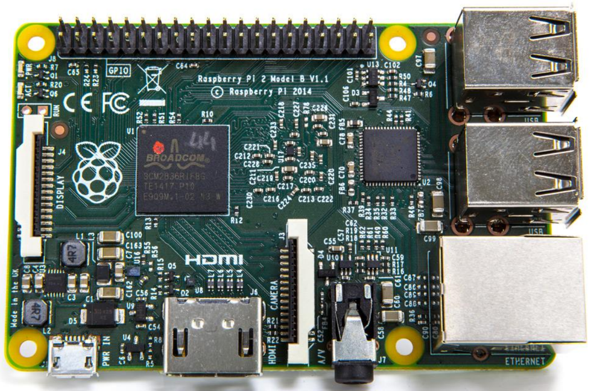
Ilustración 8: Raspberry Pi
