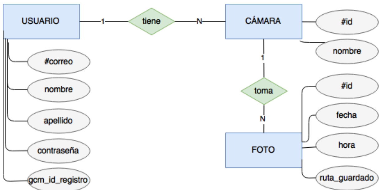
Ilustración 13: Modelo Entidad-Relación
