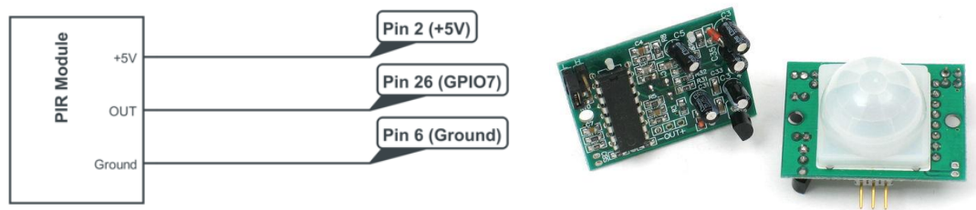
Ilustración 10: Sensor PIR
