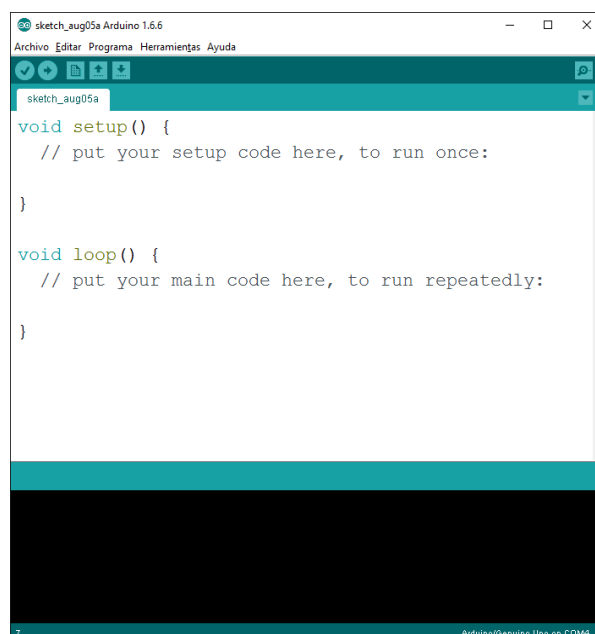
Ilustración 5: IDE Arduino
