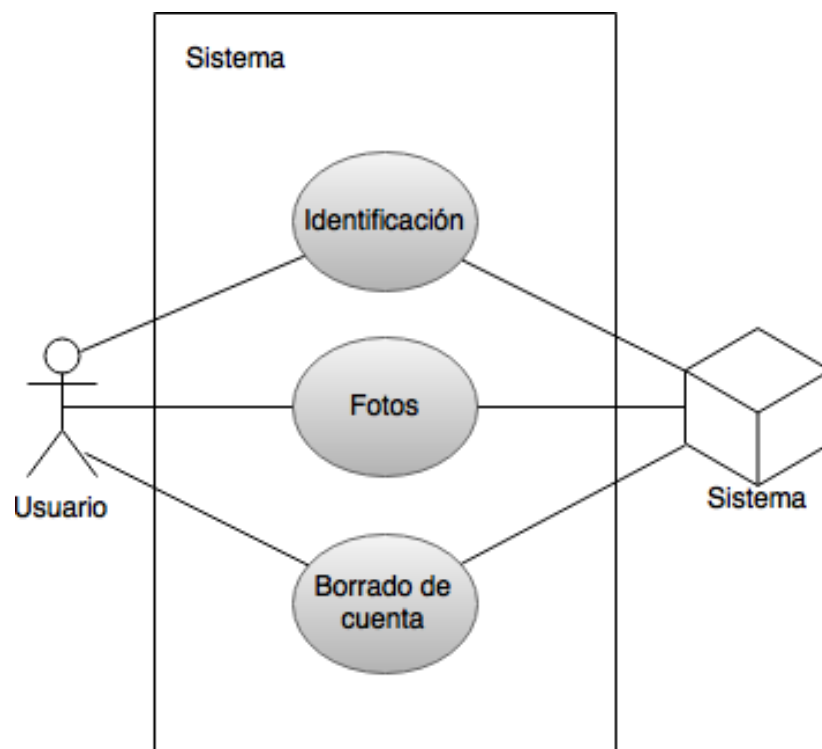
Ilustración 11: Diagrama frontera
