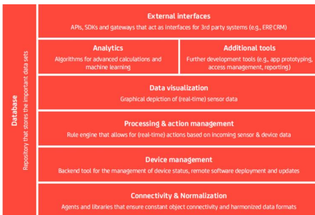
Figura 24: Funcionalidades de las Plataformas IoT (IoT Platforms: Market Report 2015-2021, 2016)
