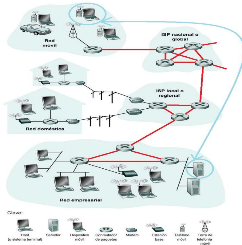
Figura 3: Principales componentes de la red. Sistemas terminales, la interacción que puede existir entre ellos (flecha azul) y el núcleo de la red (resaltado en líneas rojas) (James F. Kurose, 2010)
