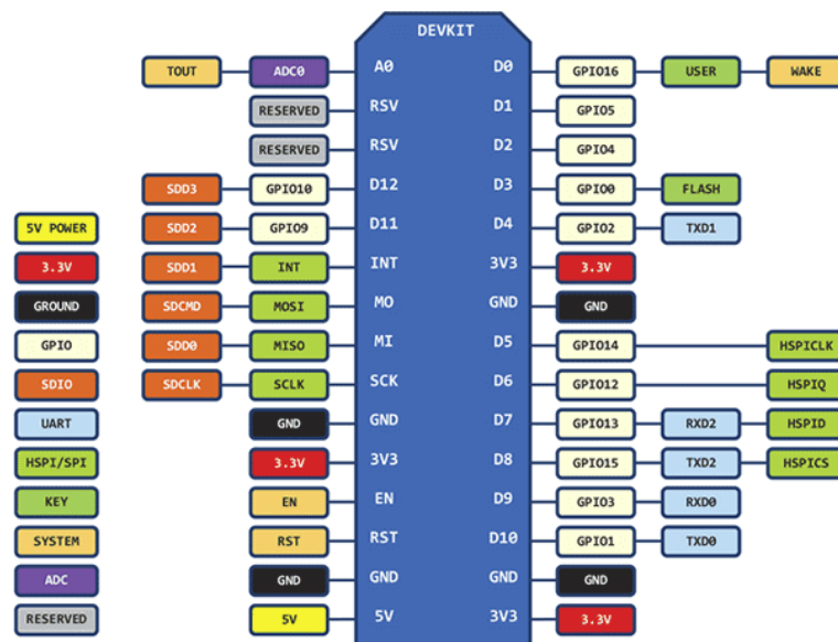
Figura 33: Pines de NodeMCU
