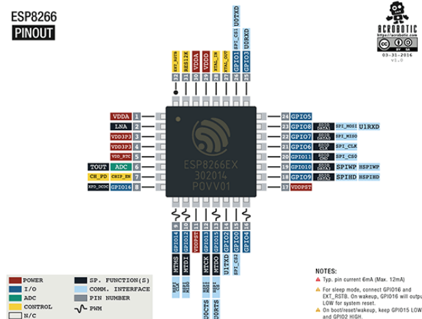
Figura 15: Disposición de los pines del ESP8266
