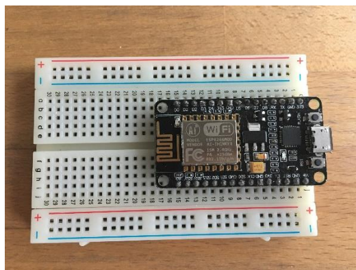
Figura 34: NodeMCU insertado en una placa de pruebas
