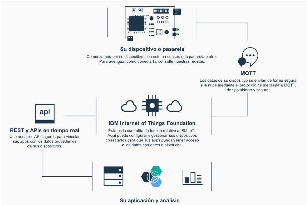
Figura 31: Esquema de funcionamiento de Watson IoT Platform
