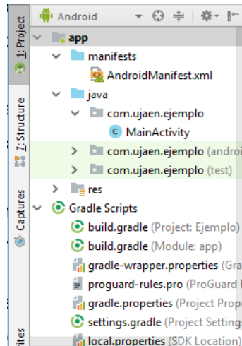
Figura 52: Vista “Android” de la ventana Project en Android Studio
