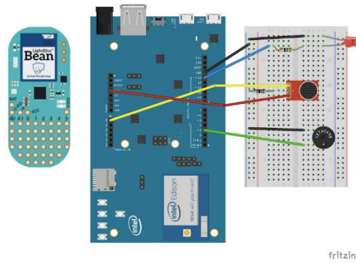
Figura 26: Sistema de seguridad desarrollado con Zetta e Intel Edison ( www.zettajs.org/projects )
