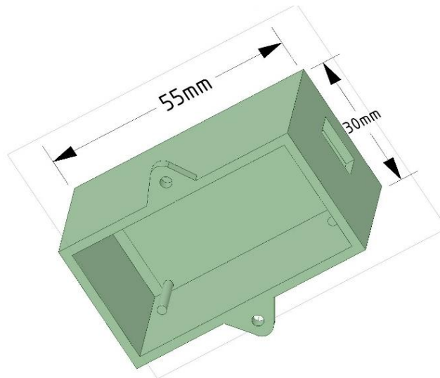
Figura 40: Pieza correspondiente a la caja de nuestra carcasa
