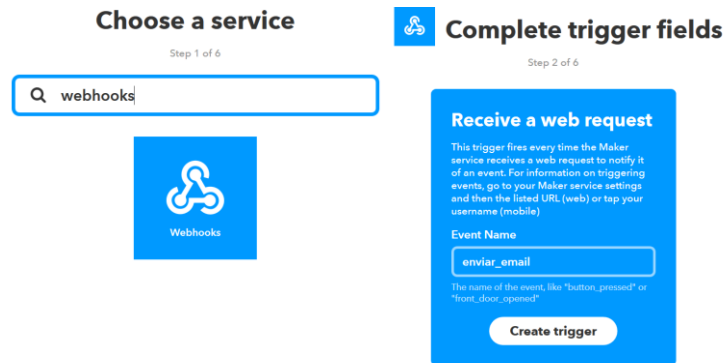
Figura 48: Configuración de la acción o evento “This” en IFTTT
