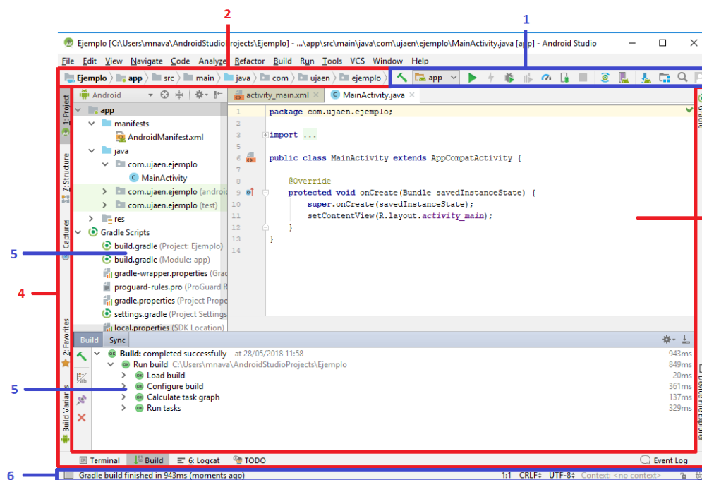
Figura 53: Interfaz de usuario de Android Studio
