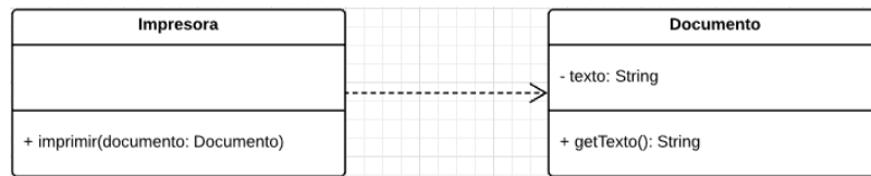
Figura 76: Ejemplo de una dependencia en UML
