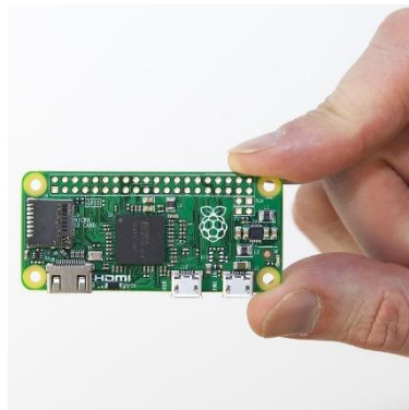
Figura 14: La nueva gama Raspberry Pi Zero, tiene un tamaño de 65 x 30 mm
