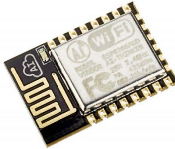
Figura 16: Módulo ESP-12 que integra un ESP8266, es similar en tamaño a una moneda
