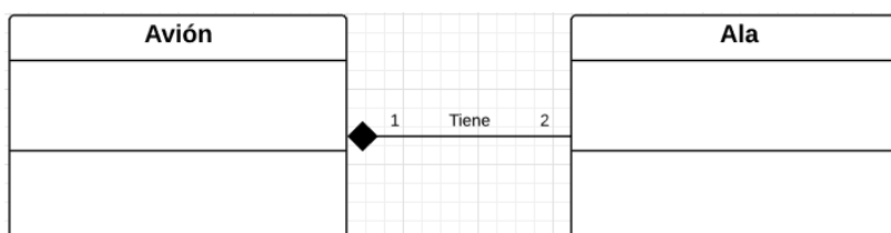
Figura 75: Ejemplo de una composición en UML
