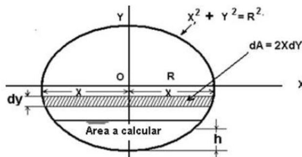
Figura 46: Corte transversal de un depósito tipo cisterna
