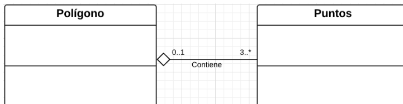
Figura 74: Ejemplo de una agregación en UML
