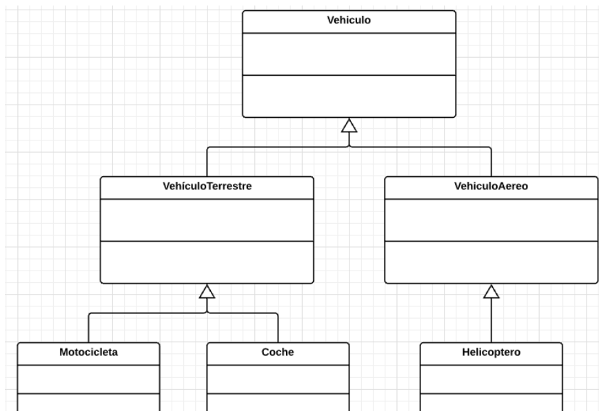
Figura 77: Ejemplo de herencia en UML
