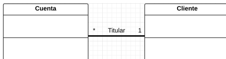
Figura 73: Ejemplo de una asociación en UML
