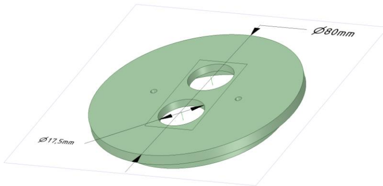
Figura 39: Pieza correspondiente a la base de nuestra carcasa
