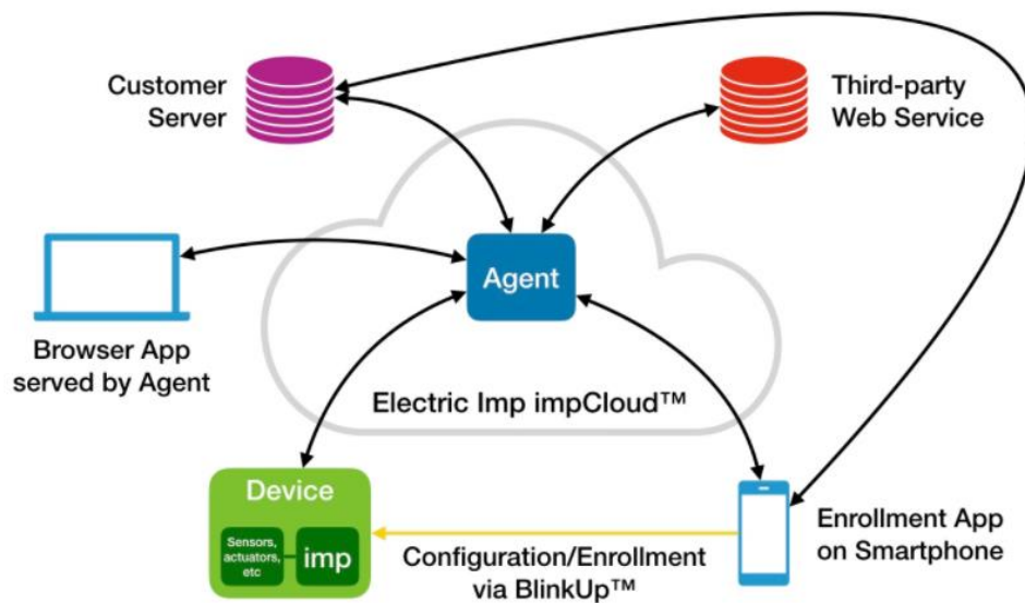
Figura 30: Esquema de funcionamiento de Electric Imp
