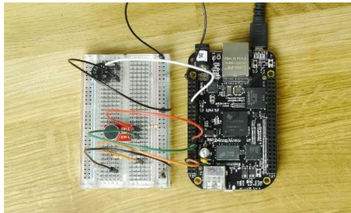
Figura 25: Sistema de seguridad desarrollado con Zetta y BeagleBone ( www.zettas.org/projects )
