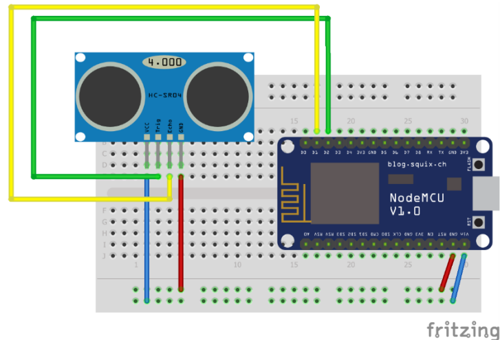
Figura 37: Esquema de conexión NodeMCU y HC-SR04
